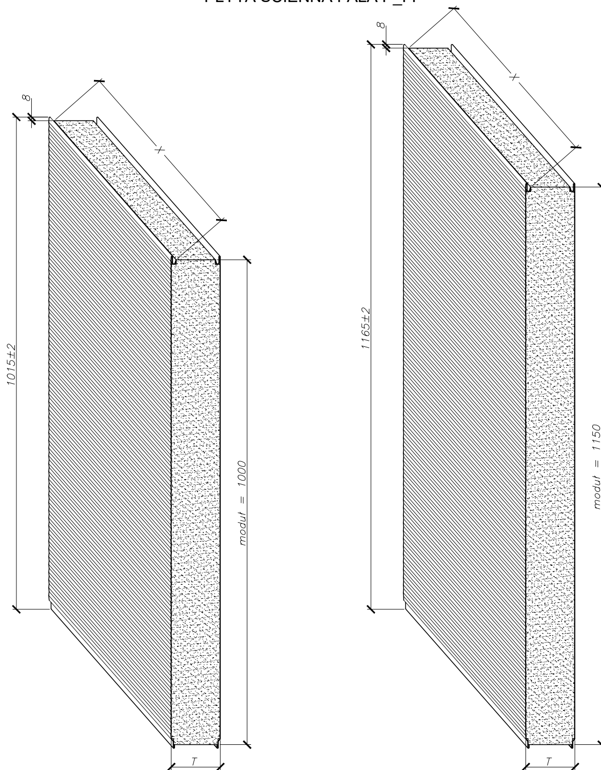
RYS. 7 PŁYTA ŚCIENNA FAŁA P_FP
