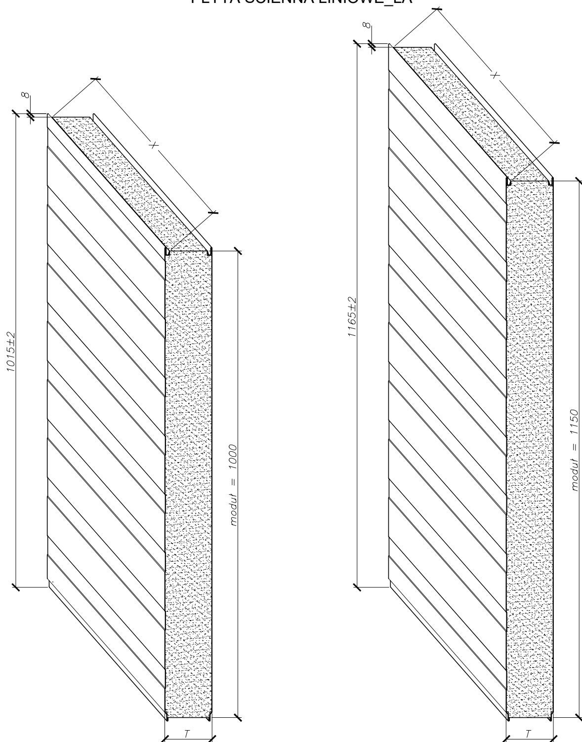
RYS. 6 PŁYTA ŚCIENNA LINIOWE_LA
