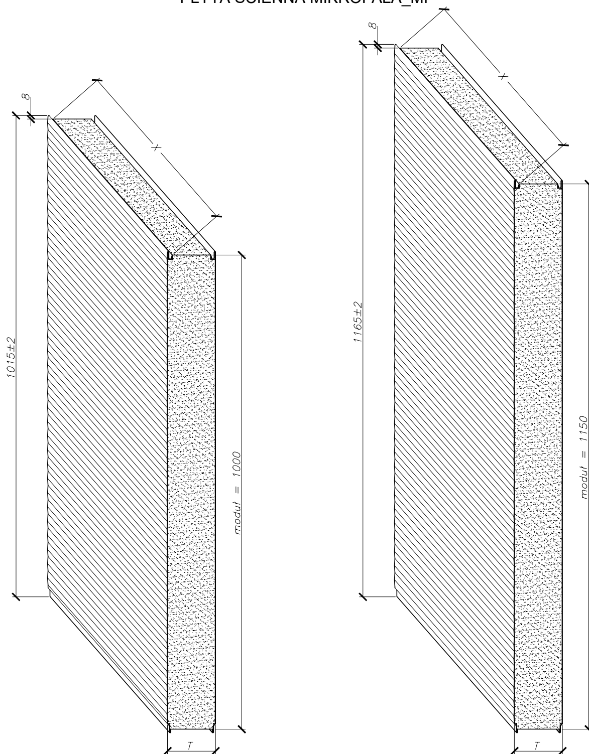
RYS. 4 PŁYTA ŚCIENNA MIKROFAŁA_MF
