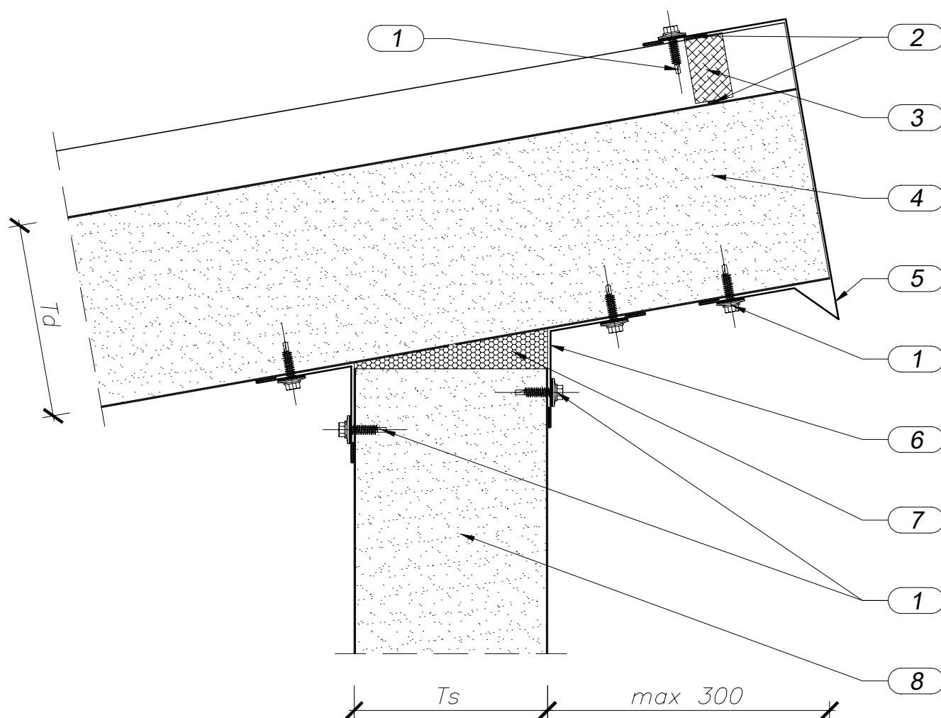
RYS. 48 POŁĄCZENIE PŁYTY ŚCIENNEJ Z PŁYTA DACHOWĄ PRZEKRÓJ PODLUŻNY wariant II
