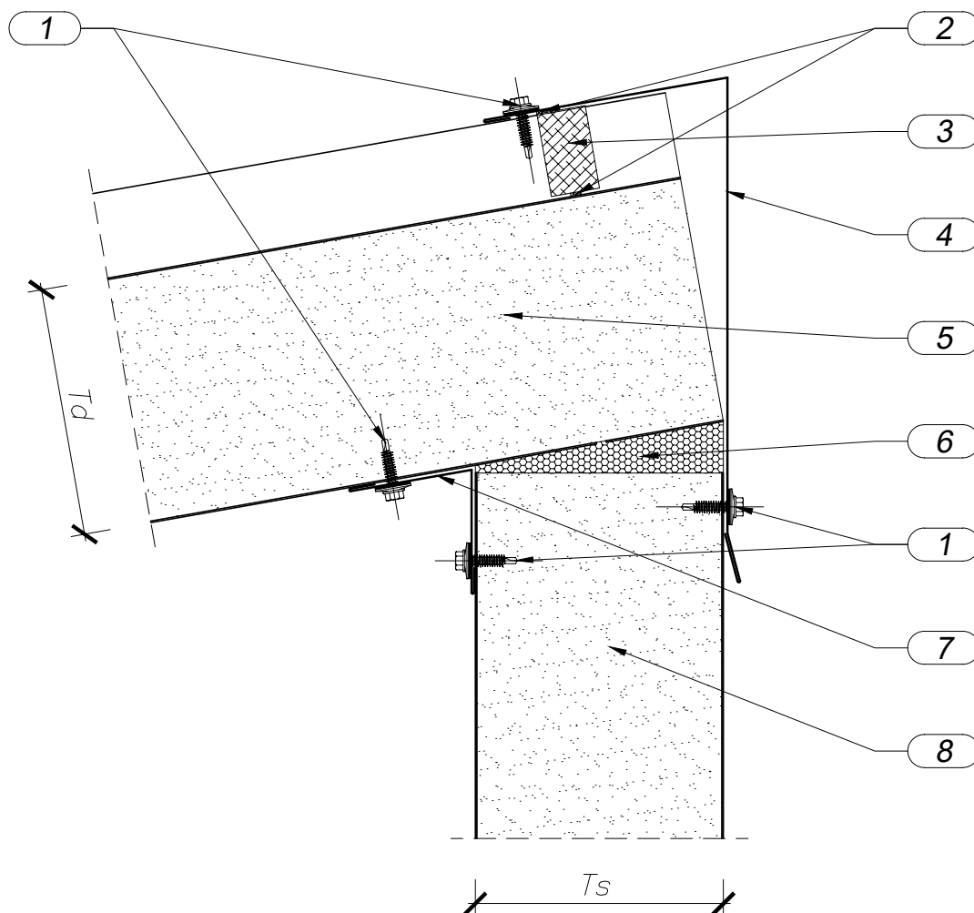
RYS. 47 POŁĄCZENIE PŁYTY ŚCIENNEJ Z PŁYTĄ DACHOWĄ PRZEKRÓJ PODLUŻNY wariant I
