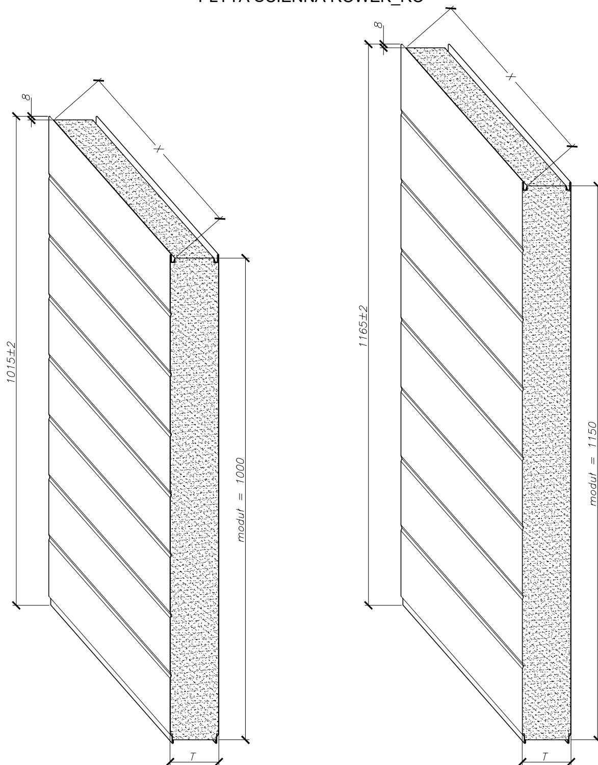
RYS. 2 PŁYTA ŚCIENNA ROWEK_RO
