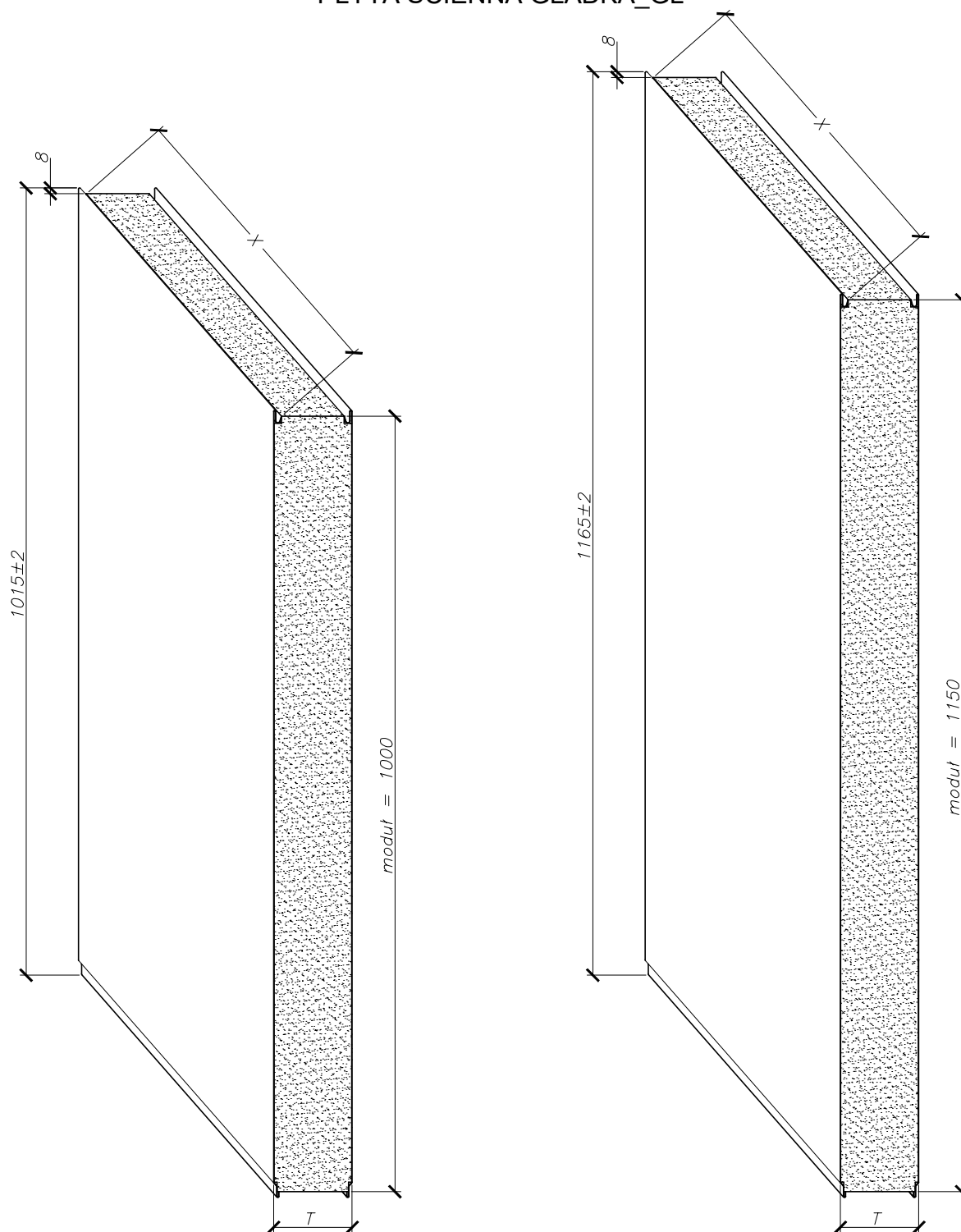
RYS. 1 PŁYTA ŚCIENNA GŁADKA_GL
