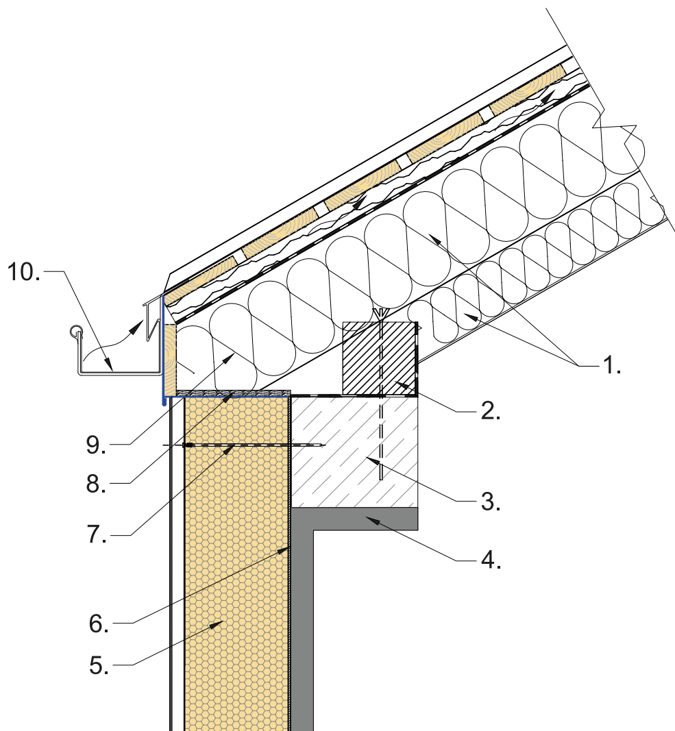
RYS. 28 STYK DACHU ZE ŚCIANĄ WRAZ Z DOCIEPLENIEM PŁYTA ALAMENTTI DESIGN ONE - Wariant 2B
