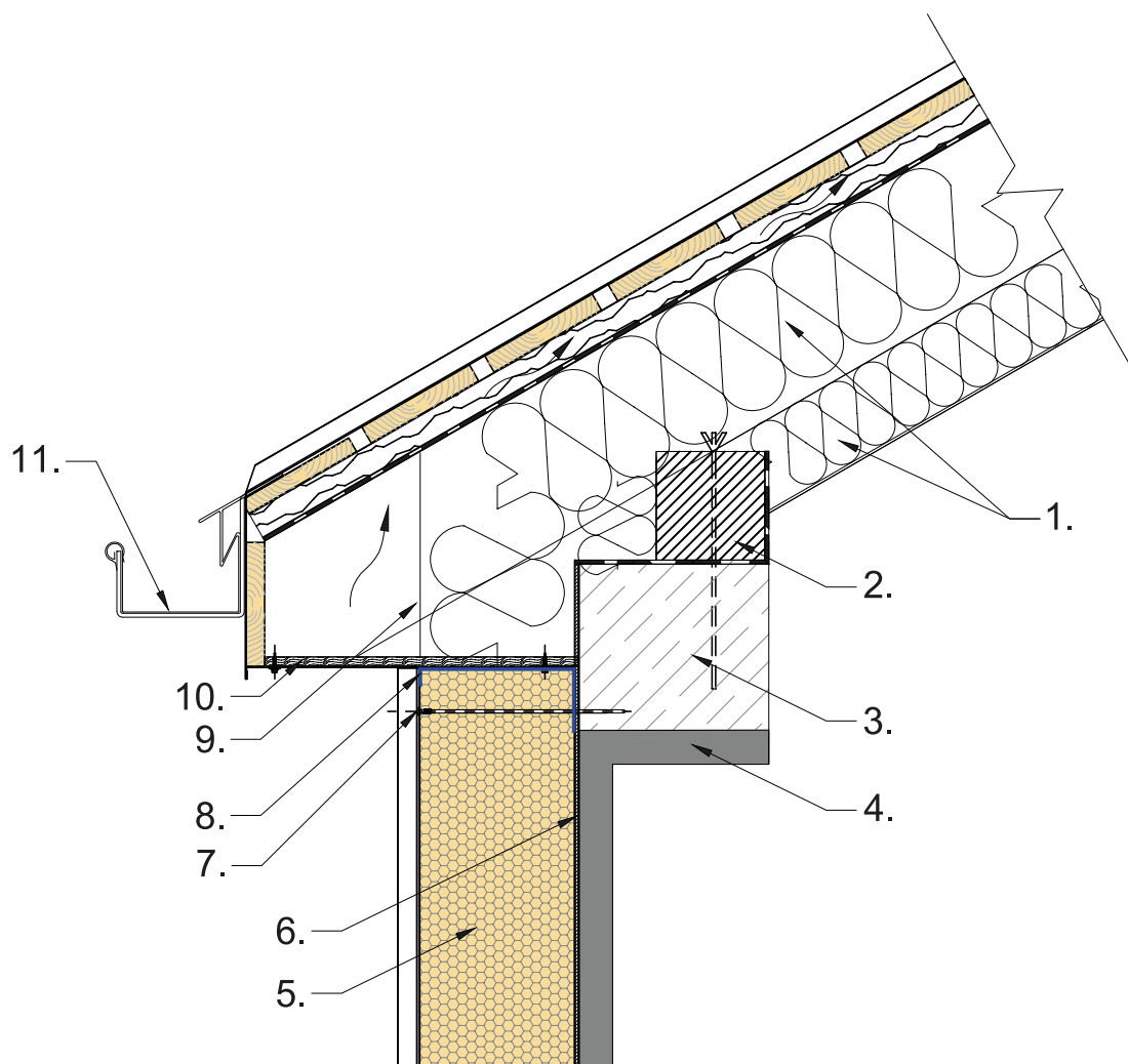
RYS. 27 STYK DACHU ZE ŚCIANĄ WRAZ Z DOCIEPLENIEM PŁYTA ALAMENTTI DESIGN ONE - Wariant 2A
